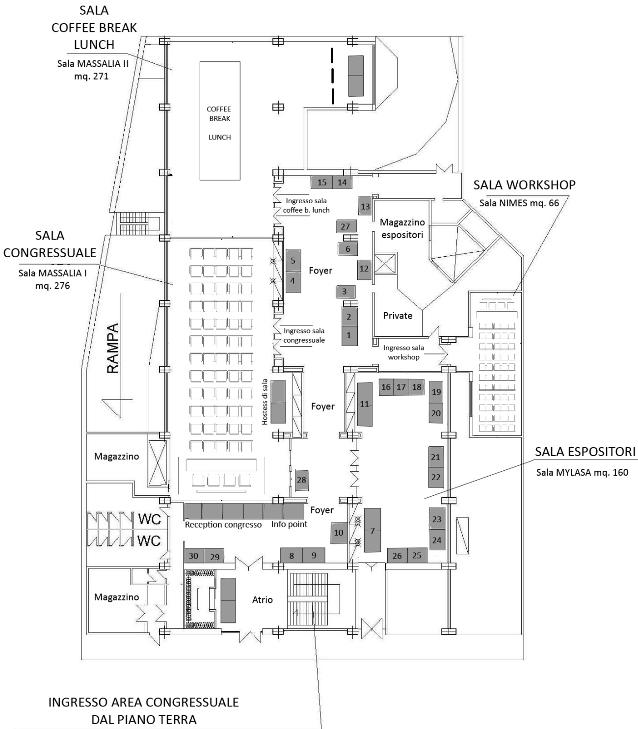
1° PIANO INTERRATO
